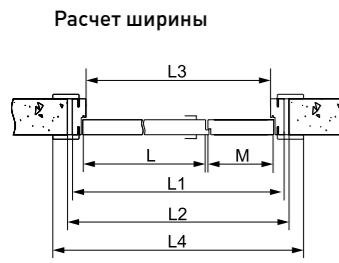
Расчет ширины
